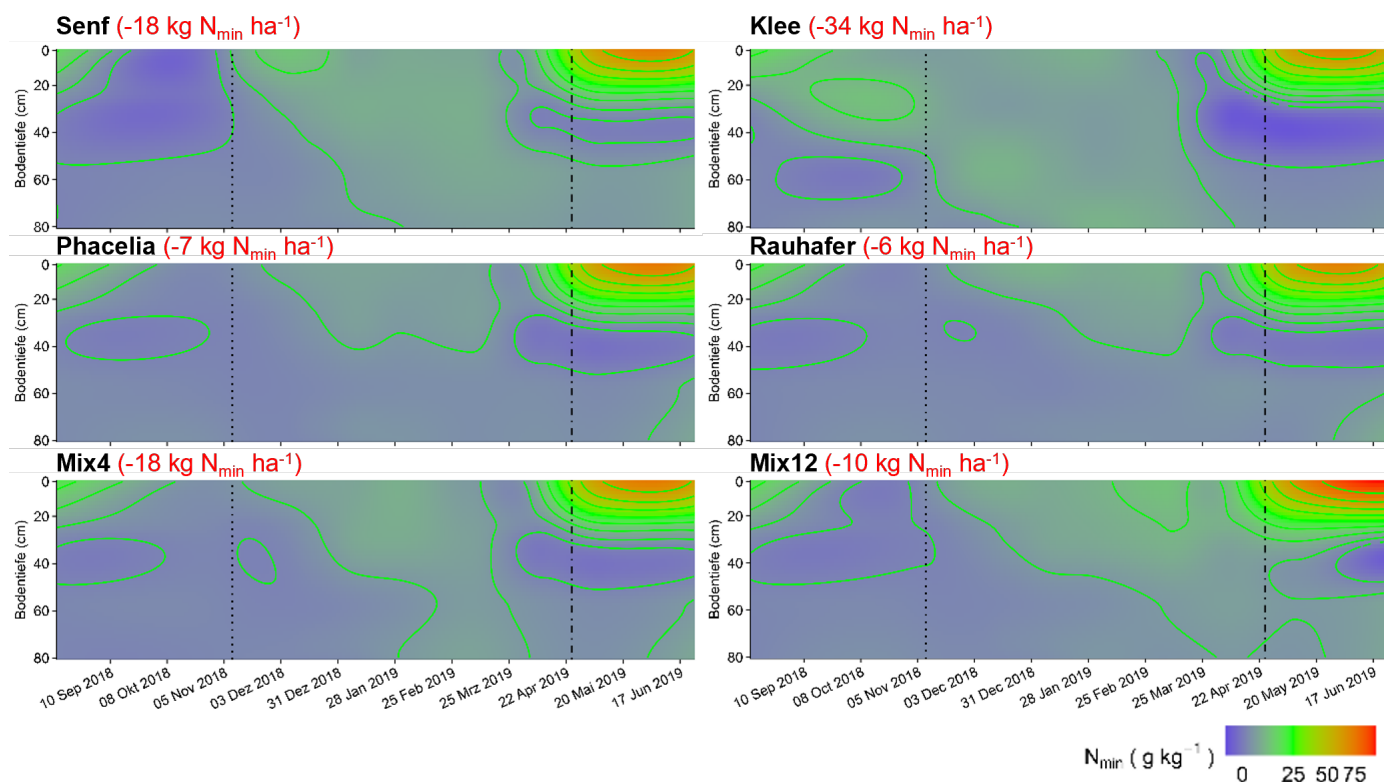
Abb. 4-4: Kontinuierliche Messungen von N_{\min} im Boden unter verschiedenen Zwischenfrüchten von Herbst 2018 bis Sommer 2019 am Standort Asendorf. Die gestrichelten Linien markieren das Absterben der Zwischenfrucht in 2018 und die Maisaussaat mit Stickstoffdüngung in 2019. Die Farben beschreiben Stickstoffkonzentrationsänderungen über die Zeit (x-Achse).
