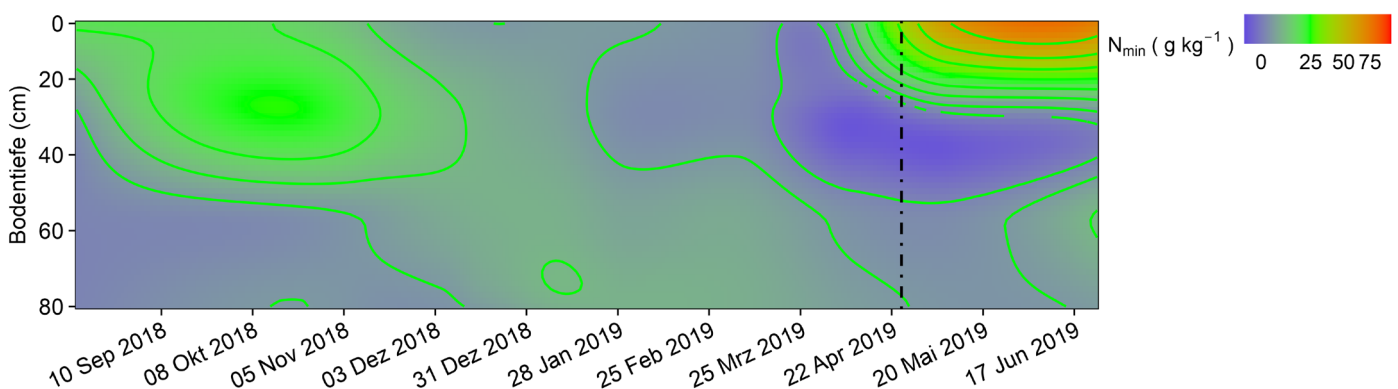
Abb. 4-3: Kontinuierliche Messungen von N_{\min} im Boden unter der Brache von Herbst 2018 bis Sommer 2019 am Standort Asendorf. Die gestrichelte Linie markiert die Maisausaat und Stickstoffdüngung. Farben beschreiben N_{\min} -Konzentrationsänderungen über die Zeit (x-Achse). Die N_{\min} -Verluste aus dem Bodenprofil summierten sich auf 102 \text{ kg ha}^{-1} bis zur Maisausaat.
